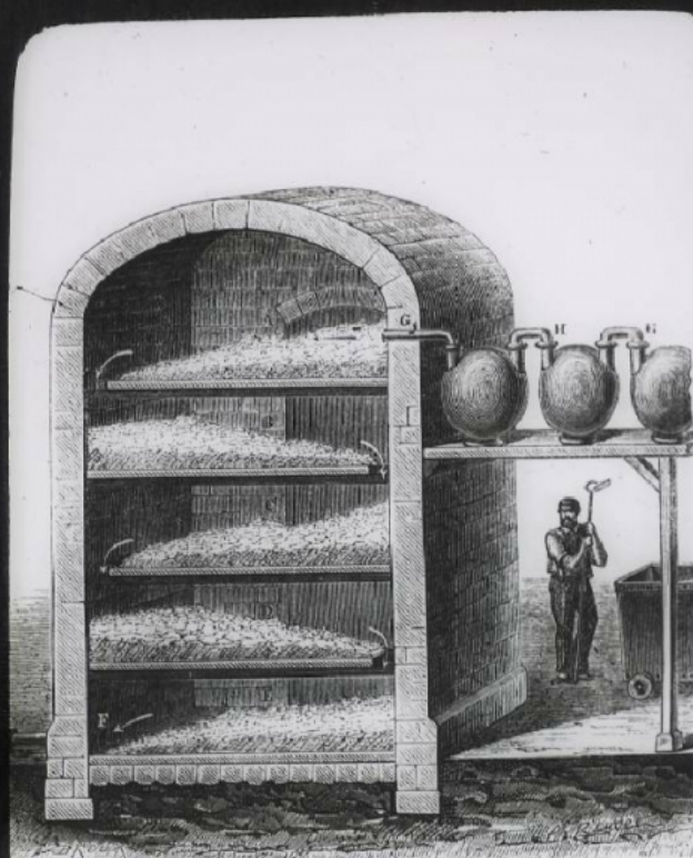
- Coupe de la chambre à blanchiment par le chlore gazeux.
