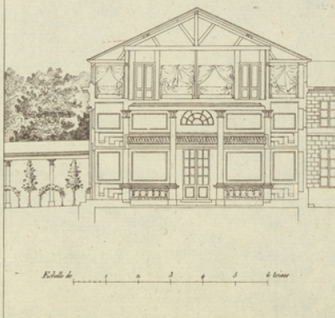
Coupe sur la largeur de la grande Salle d'Exercice
