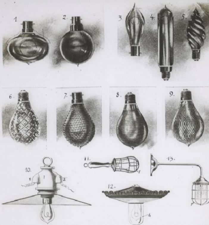
Divers Modèles de Lampes à Incandescence.
