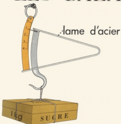
Pesons à ressort
