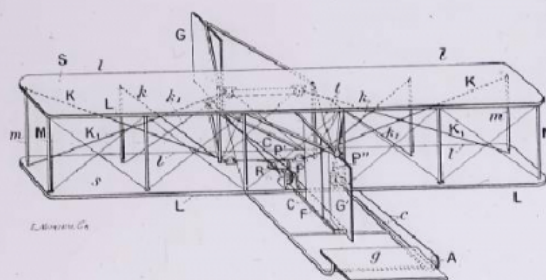
Fig. 1. - Aeroplano Wright 1907.
