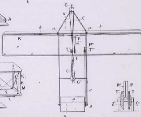
Fig. 4. - Plan.
