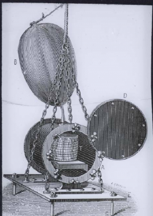
Thermomètre enregistreur de P. Regnard pour obtenir en courbe continue la température du fond des mers.
