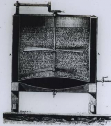
Fig. 100. — Chauffoir à vapeur des graines (C. A. 186).
