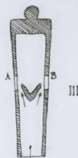
Embouchures de Tuyau sonore.
