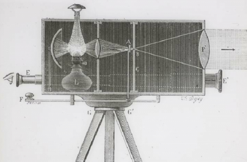
- Coupe du télégraphe optique du colonel Mangin, éclairé par une lampe à pétrole
