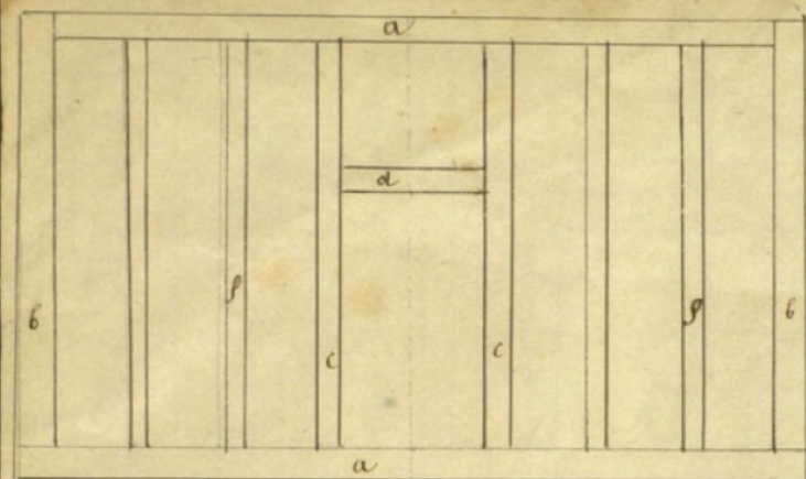
Clouon en charpente a Solliers b Poutres corniers c Poutres d'assise d Linteau f Montants ou poteaux d'emplissage
