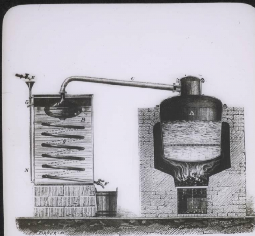
Alambic à double fond pour la distillation des marcs de raisin.
