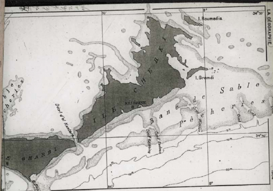
FIG. 5. — CARTE DES « OUEDES » MARIENS DES ÎLES KERKENNA. PAR M. A. ALLEMAND-MARTIN.
