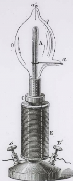
Fig. 632. — Cuf de De La Rive.
