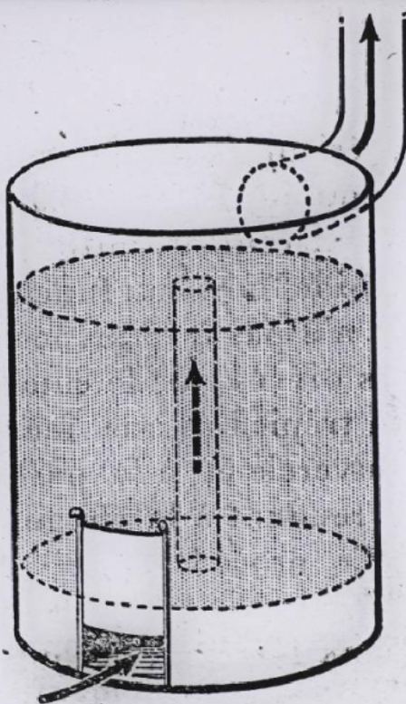
- Fourneau à sciure de type commercial.
