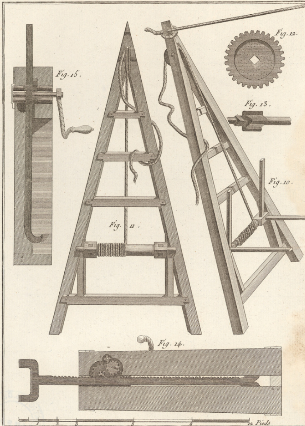
Sculpture, Instruments qui servent à monter le Marbre. Benard Dircvit. 55.
