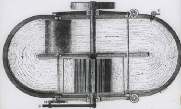
Coupe de la pile défileuse.
