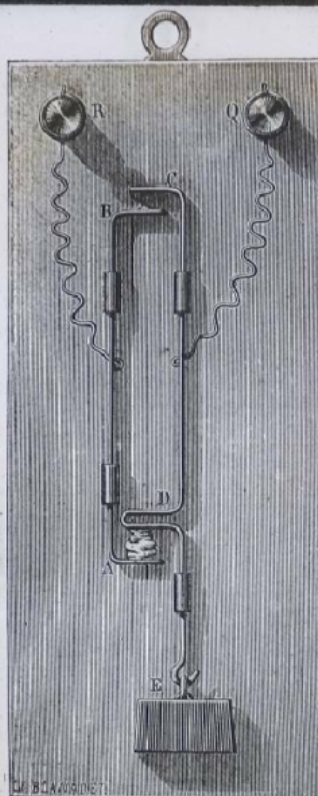
Fig. 145. — Avertisseur électrique pour incendie.
