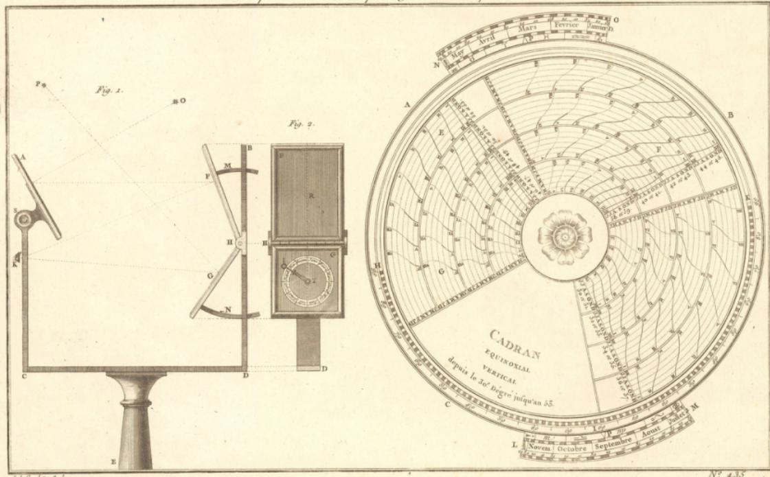
Machine pour observer le passage des Astres par le Méridien.
