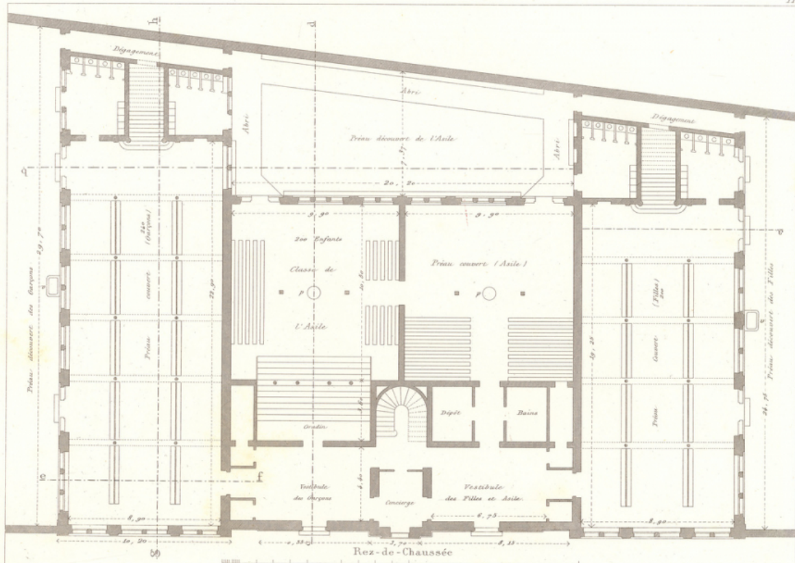
ASILE, ÉCOLE DE FILLES, ÉCOLE DE GARÇONS. Rue Keller, à Paris - M. Durand-Billion, Architecte. Paris, GARRIÈRE, Éditeur.
