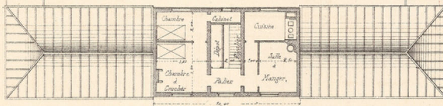
Fig 3. Plan du Rez-de-Chaussée à 0,005 pour 1 m .
