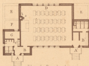
Plan du Rez-de-chaussée.
