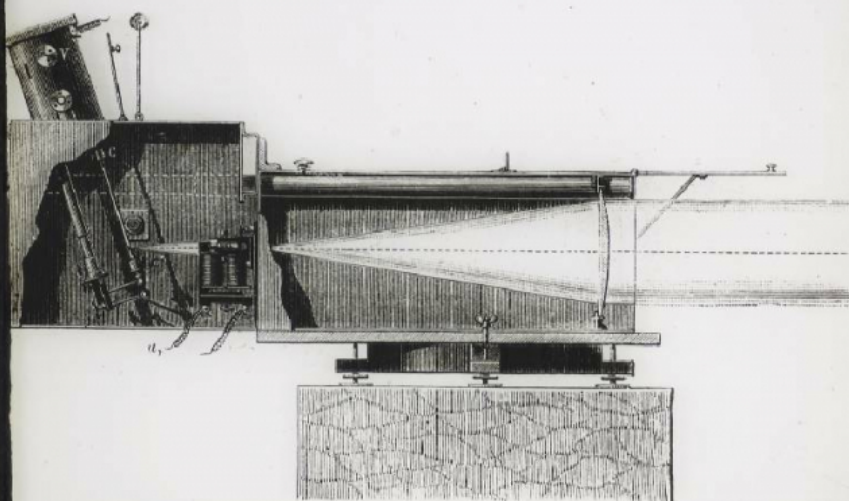
- Appareil optique ayant servi à exécuter les signaux pour la triangulation entre l'Espagne et l'Algérie (Éclairé par l'arc voltaïque).
