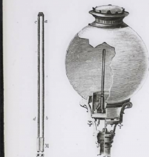
Fig. 310. Fig. 311. — Globe pour l'éclairage élec- trique par les bougies Jablochkoff.
