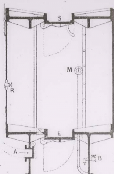
Coupe longitudinale d'une chambre d'air.
