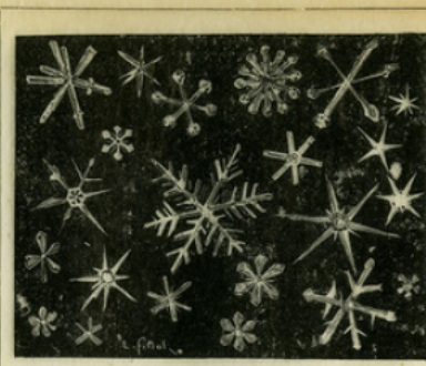
Fig. 8. — Cristaux de neige.
