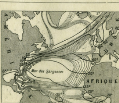
Fig. 11. — Courants marins et isothermes.
