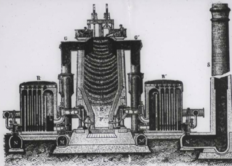
— Haut fourneau avec récupérateurs de chaleur (appareils Whitwell).
