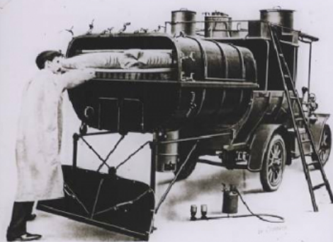
AUTOMOBILE SANITAIRE DE DION-BOUTON GONIN (L'étoffe tirée hors de son bureau a été recouverte sur ses rails. — Elle est prête à fonctionner)
