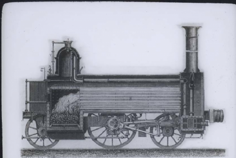
Coupe longitudinale d'une locomotive.
