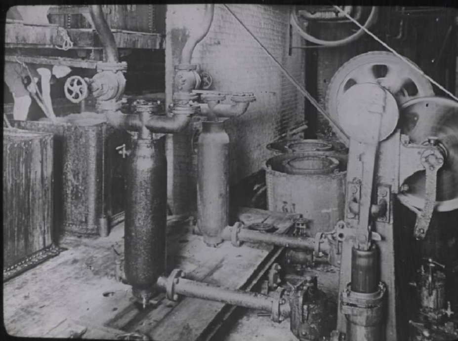
574/31 Cubes de lavage avec pompe de circulation
