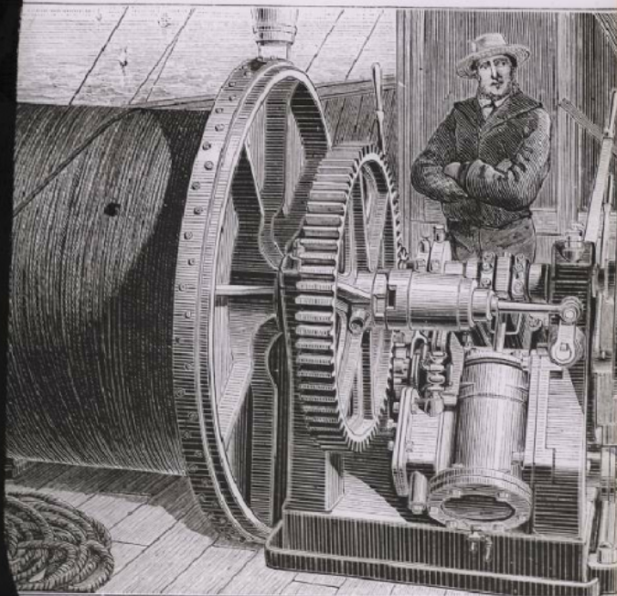
Treuil pour enrouler le câble d'acier (d'après une photographie).
