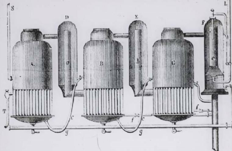
Appareil à triple effet pour l'évaporation des sirops.
