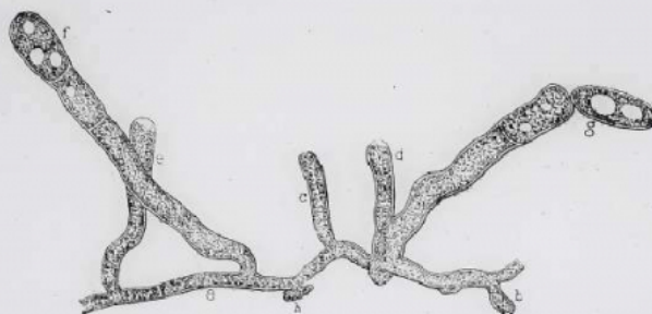
Préparation recueillie sur des grains de raisin, montrant tous les organes de l'E. Tuckeri. — a : mycélium. — b : un filament fructifère commençant à pousser. — c : filament dans lequel on ne voit encore aucune cloison. — d , e : états plus avancés, les cloisons sont formées. — f : conidiophore entièrement développé. — g : la conidie, presque entièrement détachée, n'est adhérente que par un point. — h : suçoir. — Gross. 400/1.
