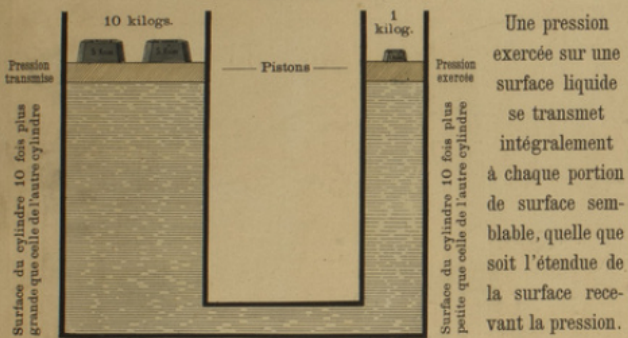
Principe de la Presse hydraulique.
