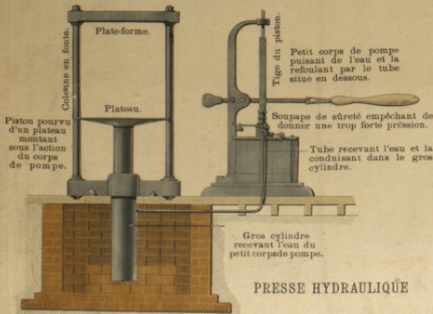
Principe de la Presse hydraulique.
