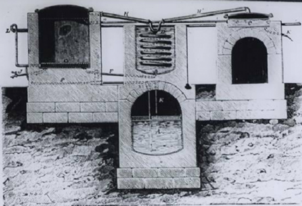
Fig. 1. — Coupe de l'appareil de M. Deiss pour l'extraction des huiles au moyen du sulfure de s.
