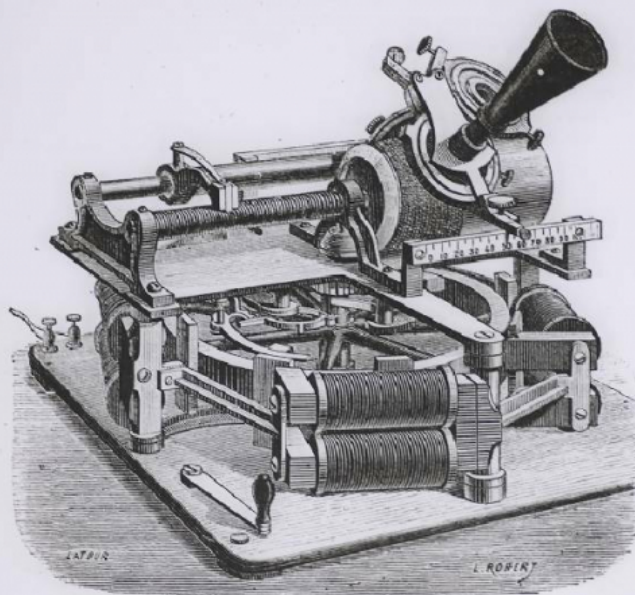
— Phonographe (nouveau modèle). ( La lumière électrique , 4 février 1888.)
