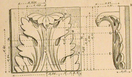
Fig. 24. — Feuille d'acanthé. (Élévation.)
