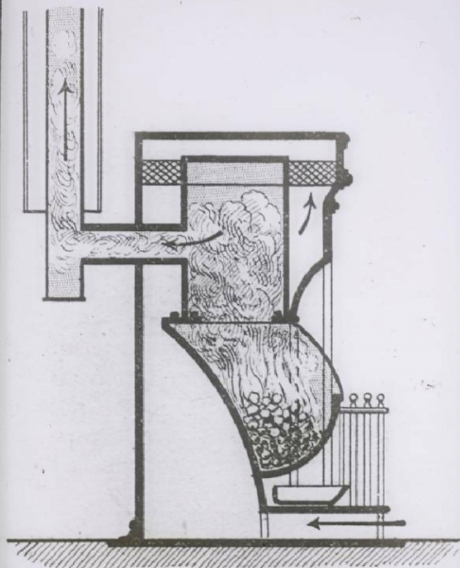
- Cheminée prussienne.
