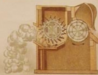
Corte ó sección de una despepitadora
