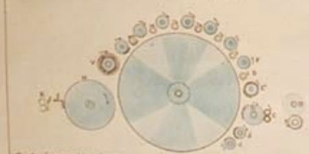
Corte ó sección de una carda
