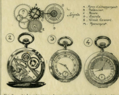
Fig. 9. — 1) Le mécanisme des montres est constitué par la détente lente et régulière du grand ressort au moyen de la roue d'échappement : celle-ci est commandée par une ancre dont le va-et-vient est produit par le balancier. — 2) Intérieur d'une montre. — 3) Cadran ordinaire. — 4) Cadran nouveau comptant vingt-quatre heures.
