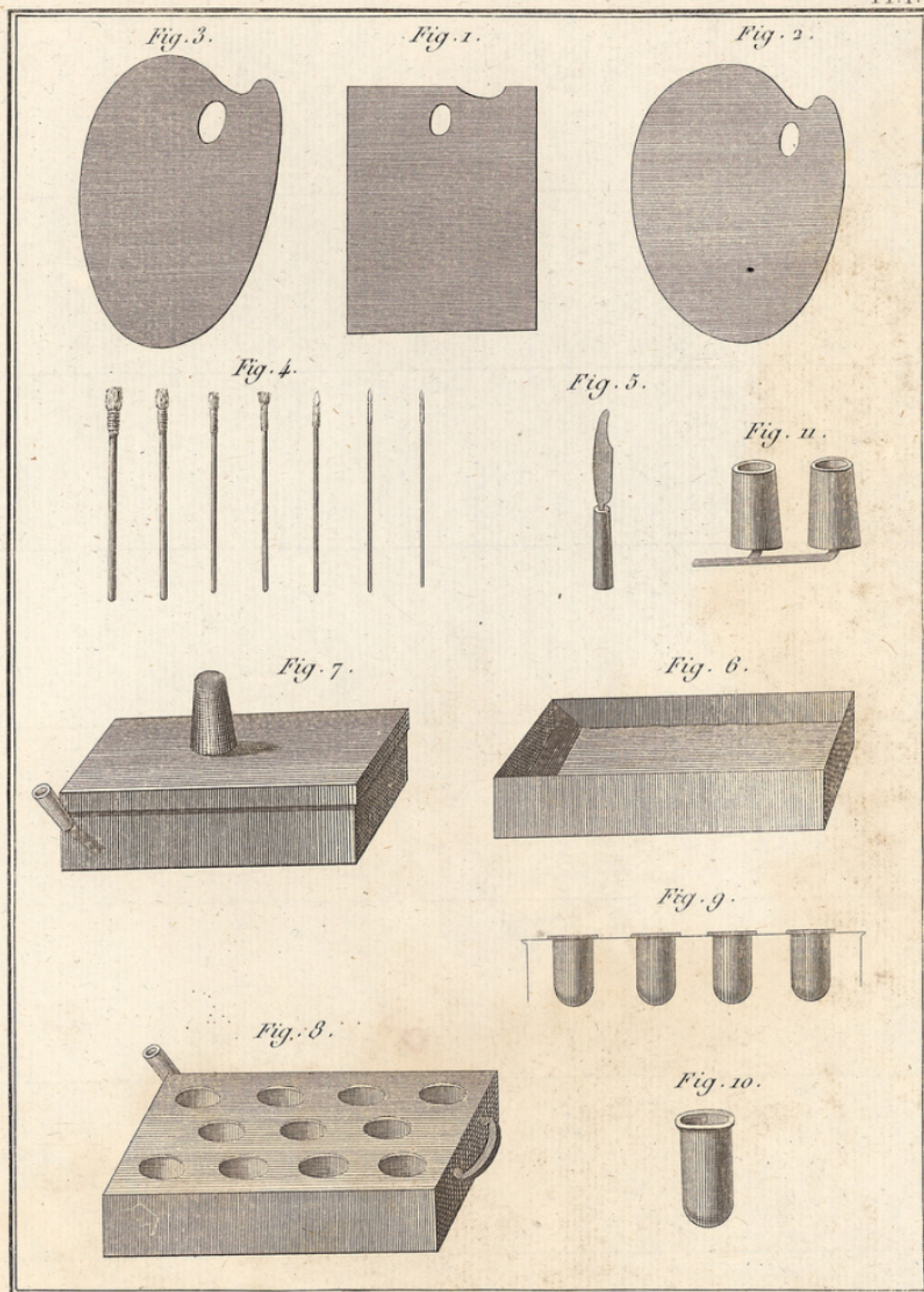
Peinture. Ustensiles de la Peinture à l'Encaustique.
