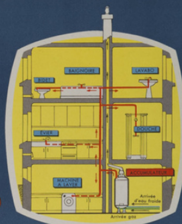
Centrale "eau chaude" d'un pavillon
