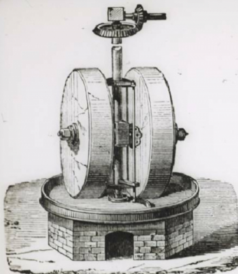
— Machines à écraser les graines et fruits alimentaires.
