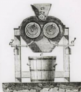
— Concasseur des graines oléagineuses.
