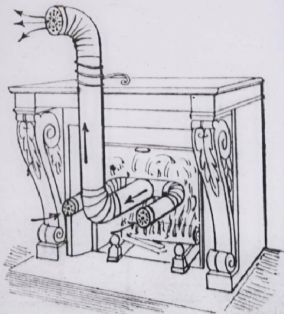
Récupérateur de chaleur de fortune construit avec de de poêle.
