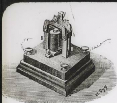
— Relais récepteur du télégraphe Baudot.
