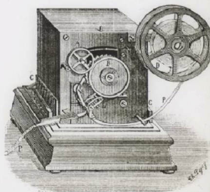
Le récepteur-imprimeur Baudot.
