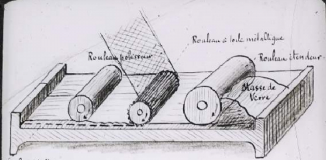
Fabrication du vene armé.
