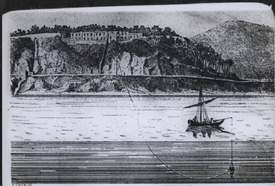
Expérience de la mesure de l'intensité lumineuse dans les eaux exécutée à Monaco en mars 1890.
