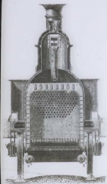
Coupe transversale par la boîte à feu.
