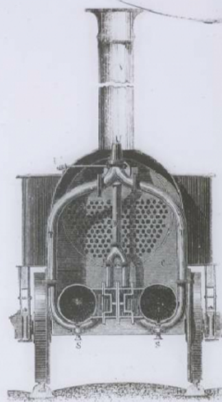
Coupe transversale par la boîte à fumée.
