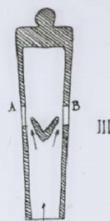
Embouchures de Tuyau sonore.
