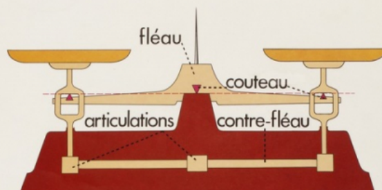
Schéma de la balance
