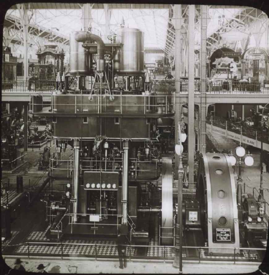
13 Machine Siemens et Halske Boyr. 1900
